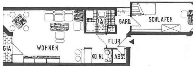
Grundriss
